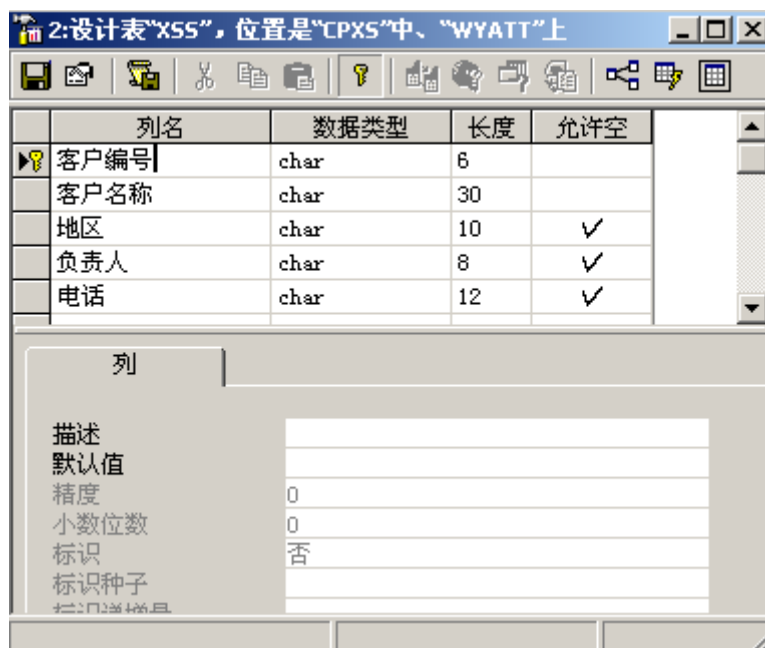
图1.2 XSS表结构
